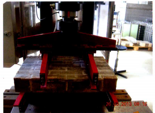
Foto 7: Buigtreksterkte gemetselde proefmuur
