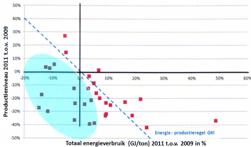
Figuur 3: Vergelijking totaal energieverbruik EEP 2009 en 2011
