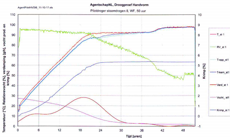
Figuur 1: Droogkarakteristiek Omgevingsluchtdrogen.
