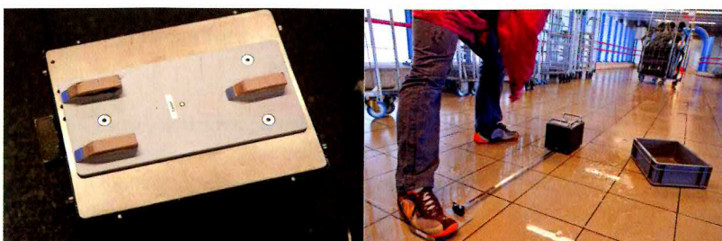
Foto 3 en 4: Opstelling en uitvoering tribometer-test
