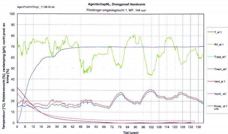
Figuur 2: Droogkarakteristiek Stoomdrogen.
